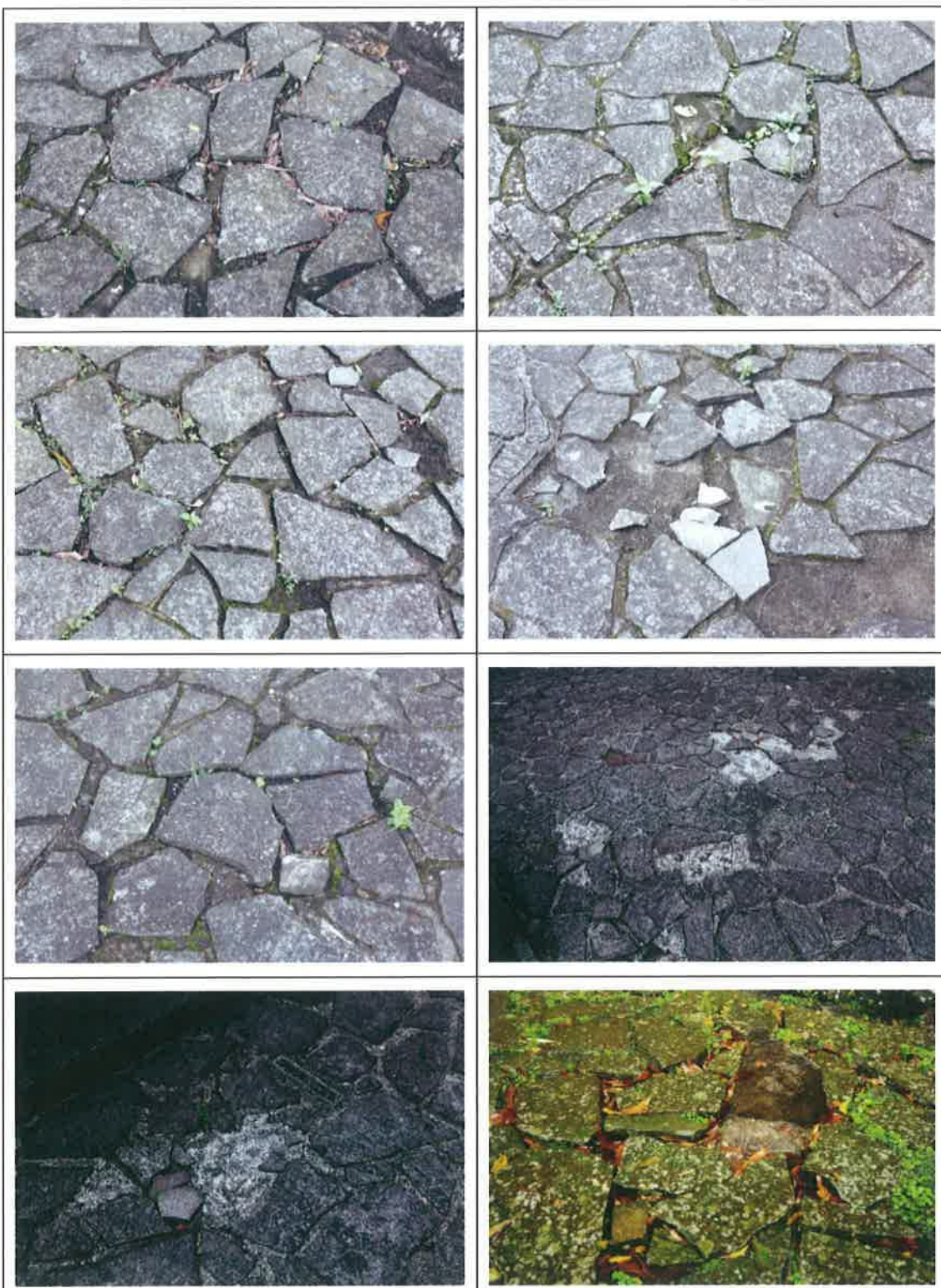
圖 95 地坪毀損情形示意圖
