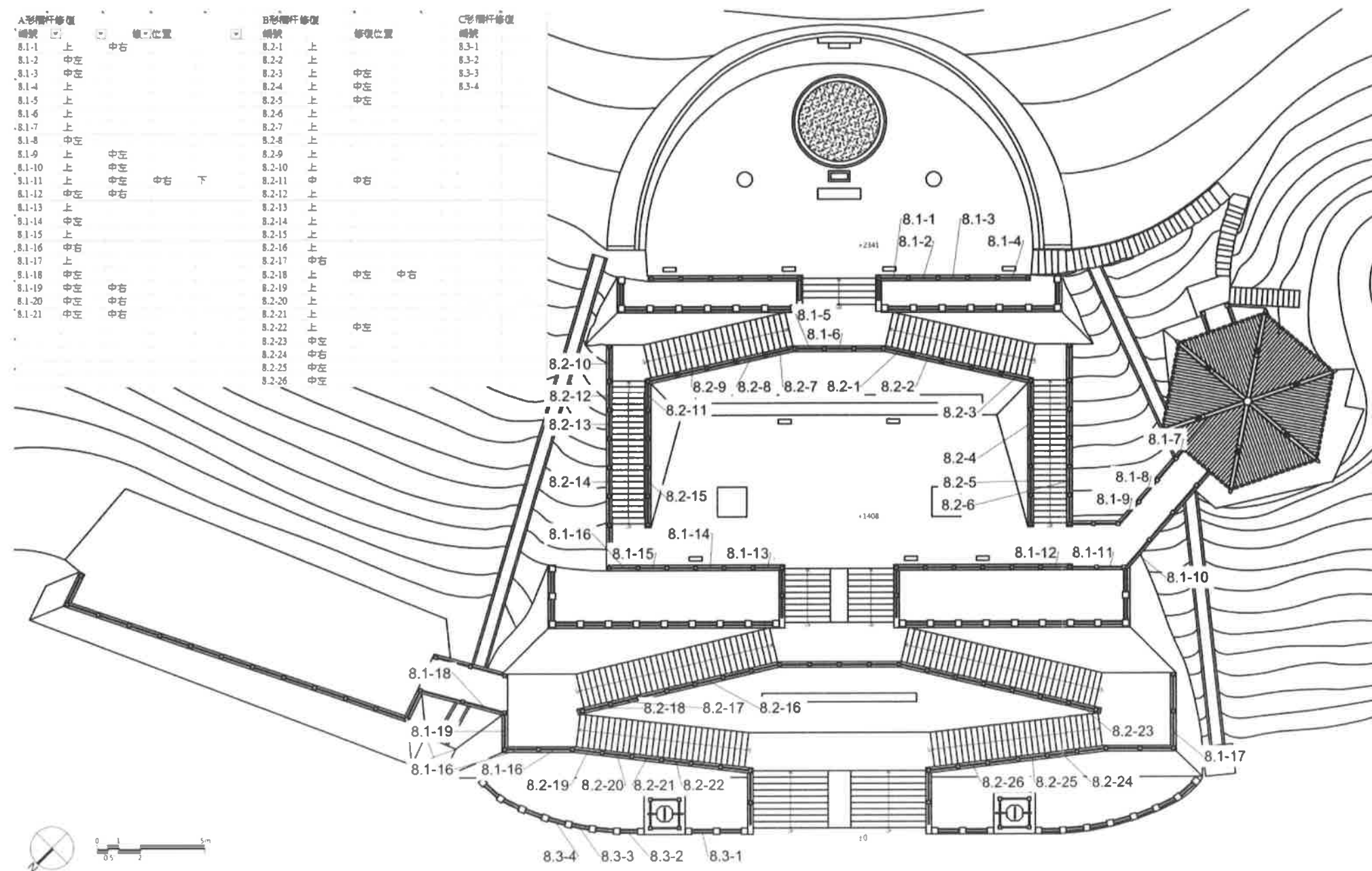
欄杆修復位置圖
