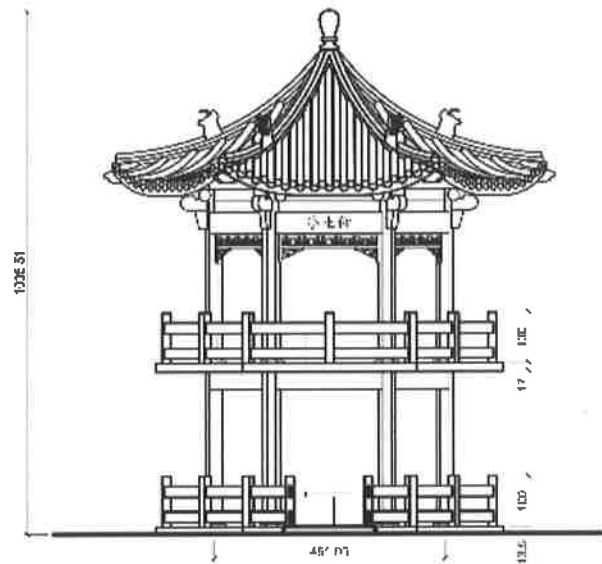
仰止亭立面圖
