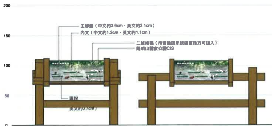
圖 104：中型資源解說牌誌設計圖。
