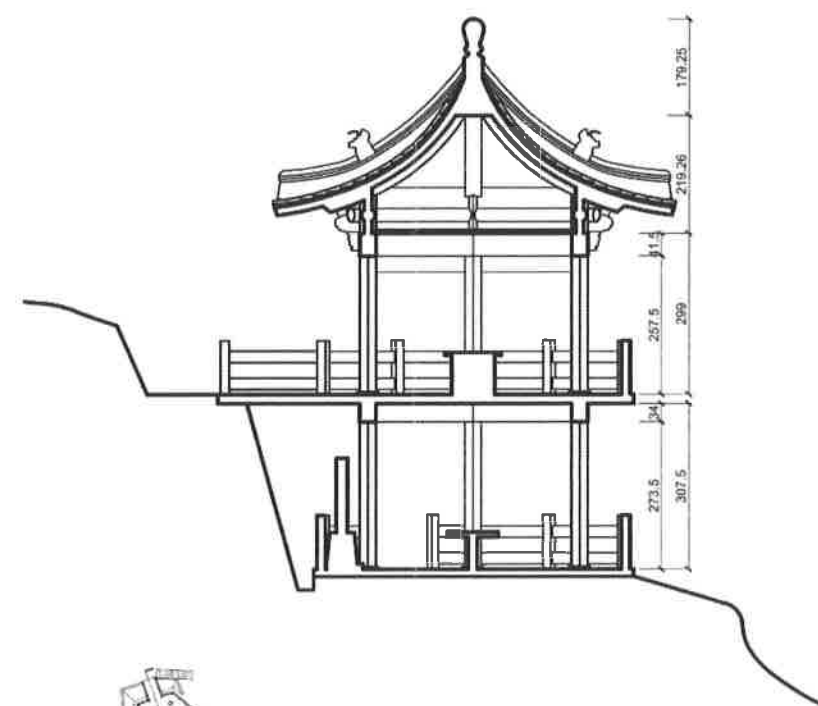
剖面圖
