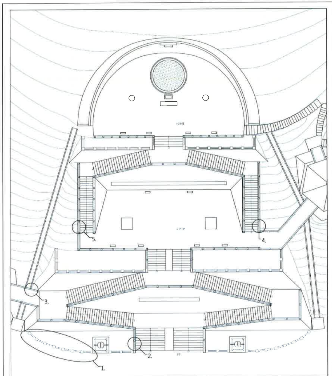
圖 90 欄杆毀損位置分布
