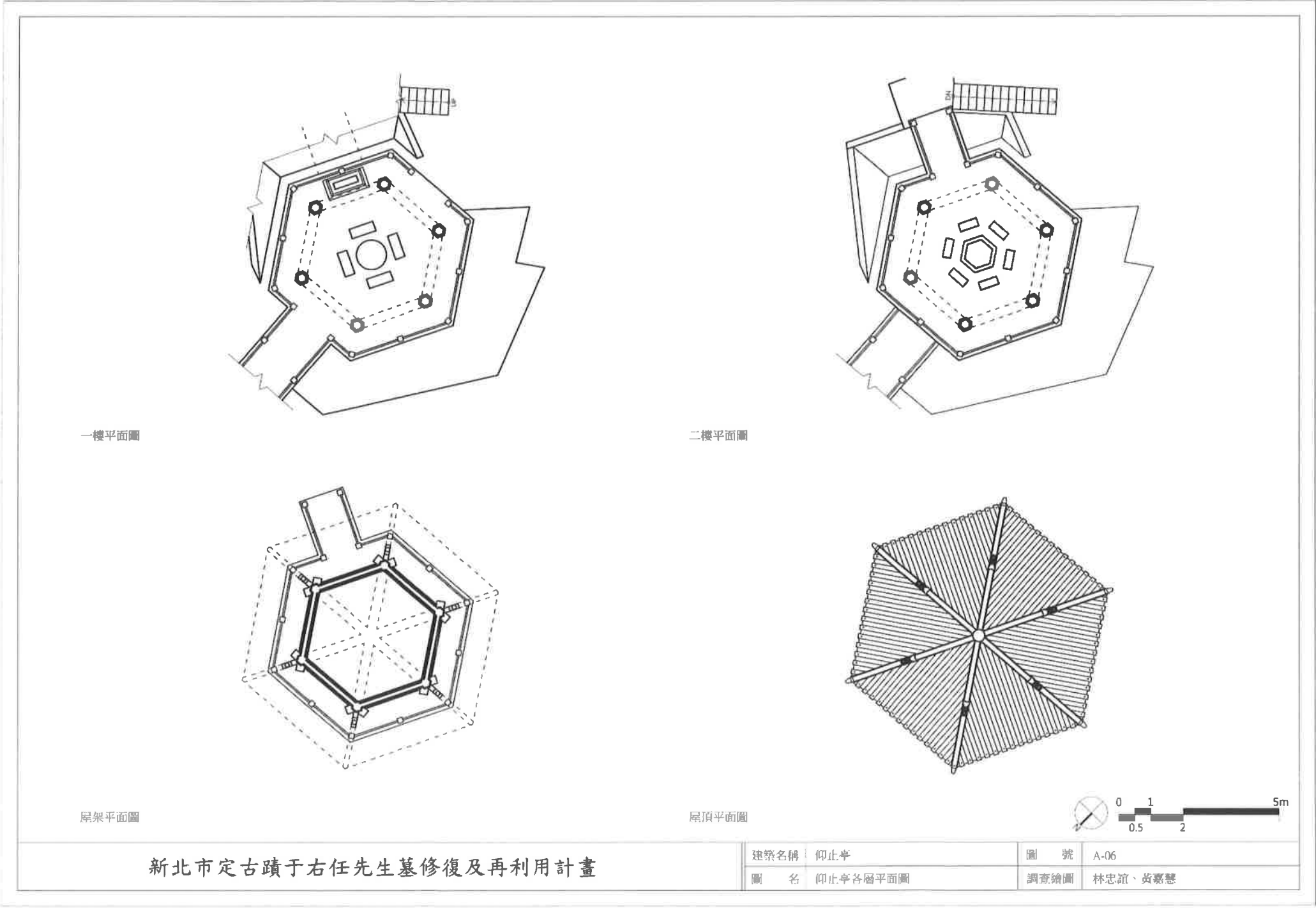
附錄二 6：仰止亭各層平面圖
