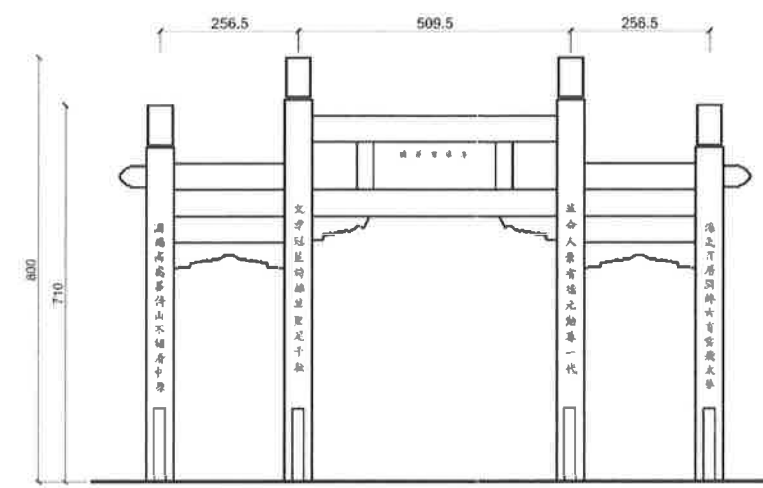
西向立面圖
