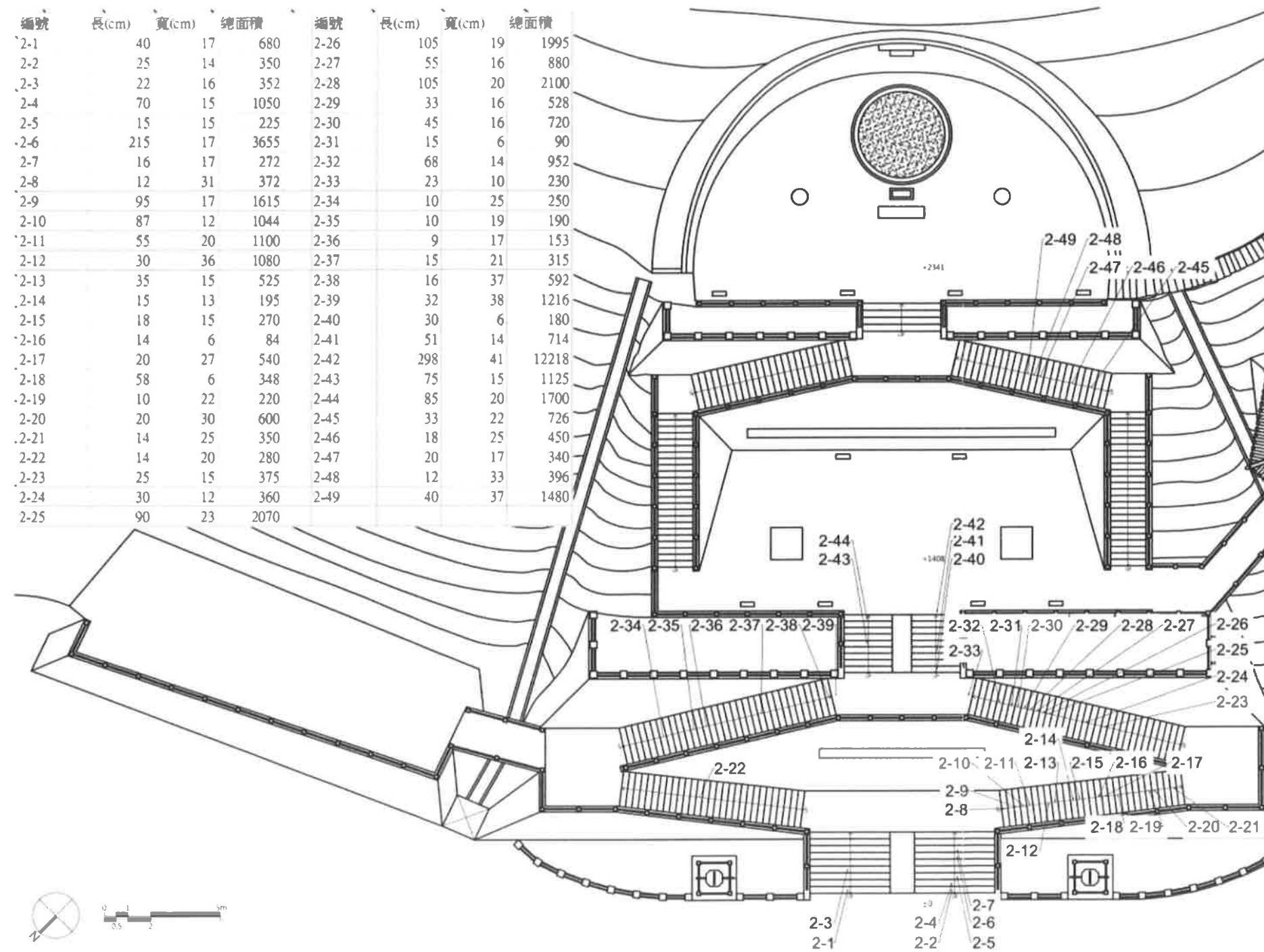
階梯修復位置圖
