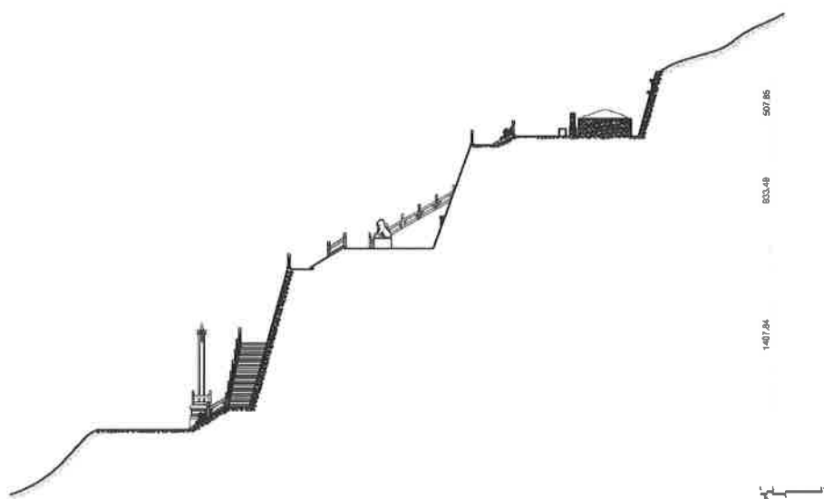
墓園剖面圖
