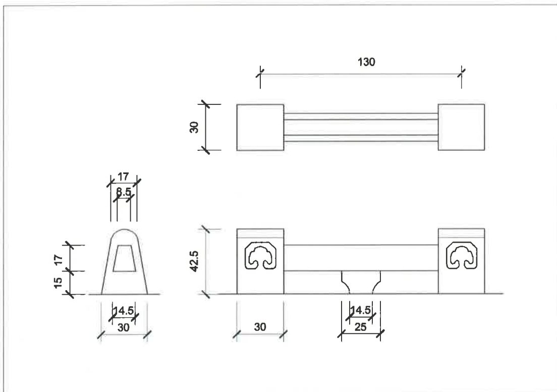
附錄二 20：須修復物件圖樣尺寸－護坡欄杆 C 樣式及尺寸大樣圖
