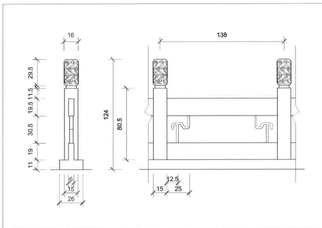
附錄二 18：須修復物件圖樣尺寸－欄杆 A 樣式及尺寸大樣圖
