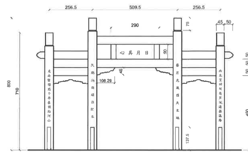
東向立面圖
