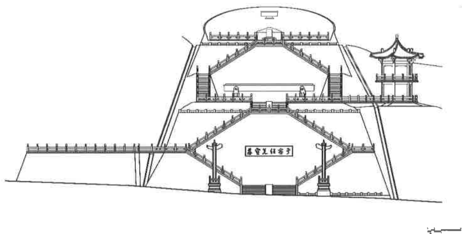
墓園立面圖
