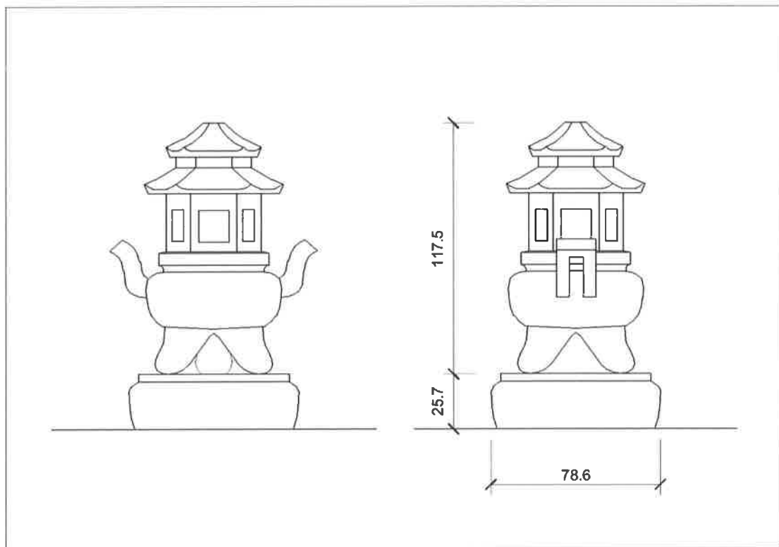
附錄二 21：須修復物件圖樣尺寸－香爐樣式及尺寸大樣圖
