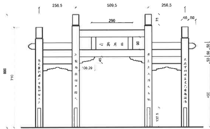
「日月其心」石牌坊立面圖
