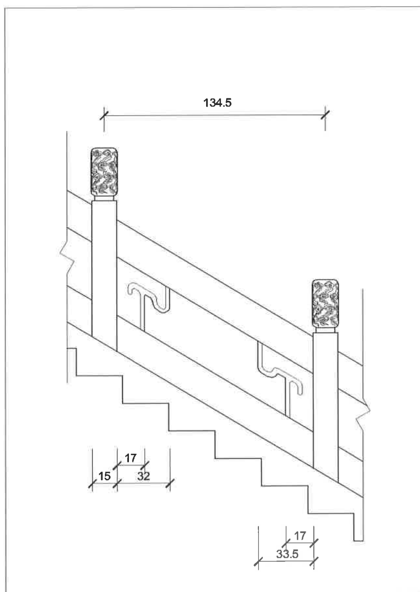
附錄二 19：須修復物件圖樣尺寸－欄杆 B 樣式及尺寸大樣圖
