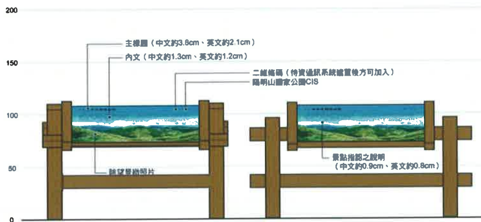
圖 103：大型資源解說牌誌設計圖。
